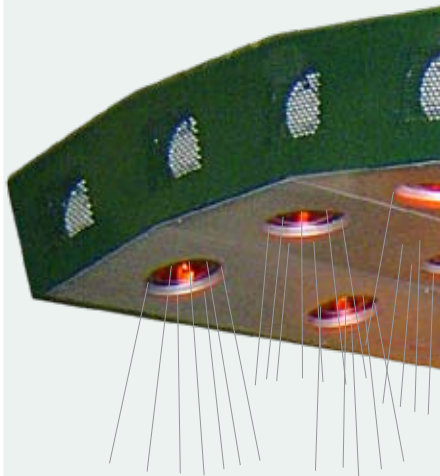
Luften från fläktarna blåses ut runt omkring glödlamporna
